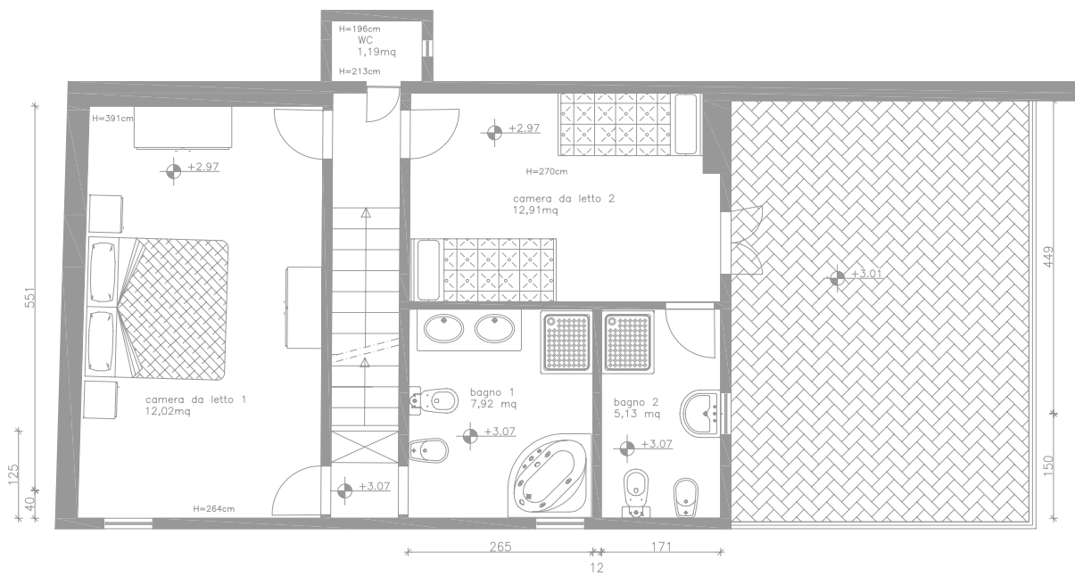
PIANO PRIMO: STATO DI PROGETTO
