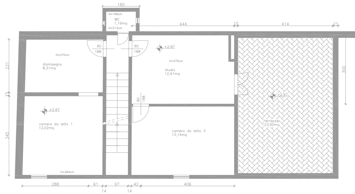
PIANO PRIMO: STATO ATTUALE
